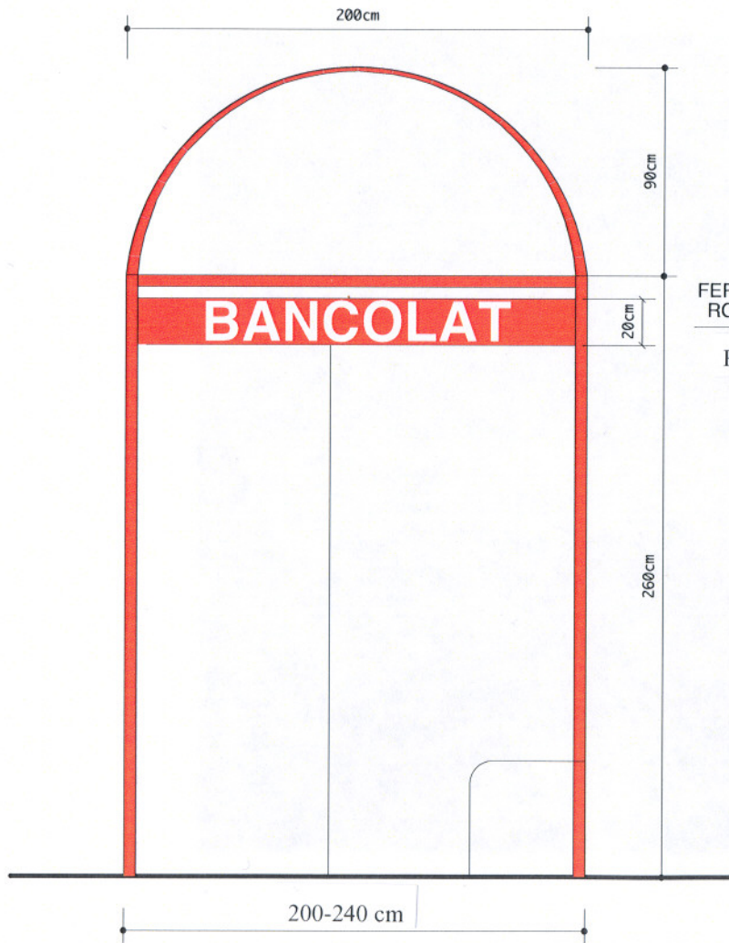
SEZ. TRASVERSALE
