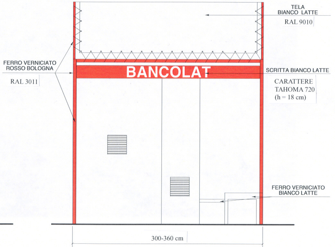
PROSPETTO
