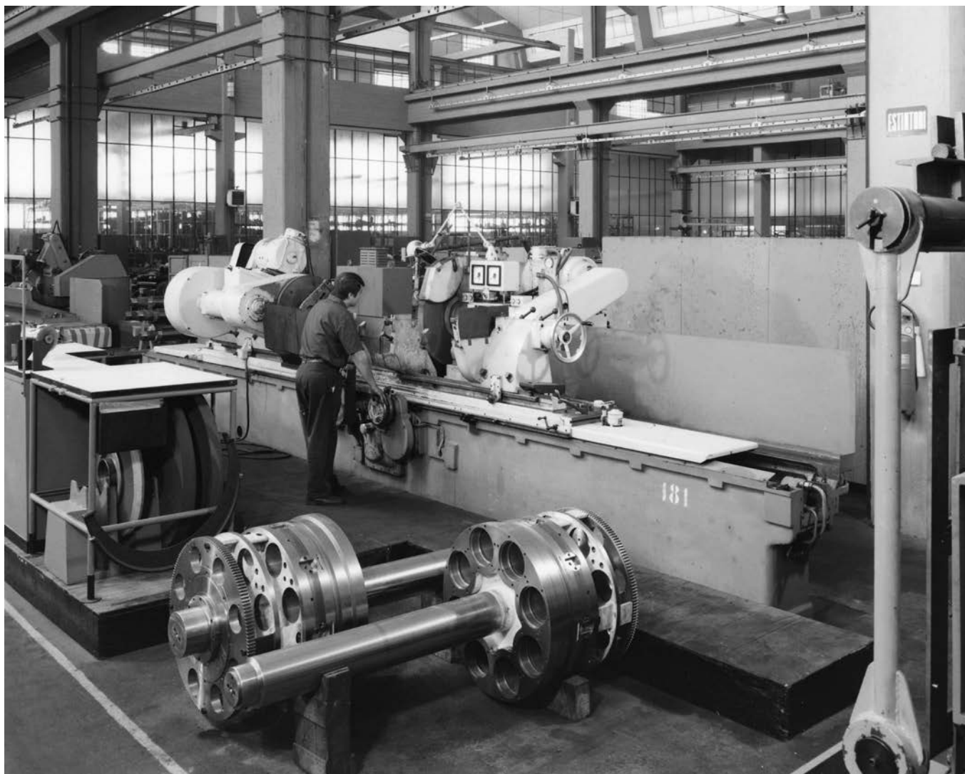
Operazione di rettifica, anni '60 Museo del Patrimonio Industriale, fondo Minganti
