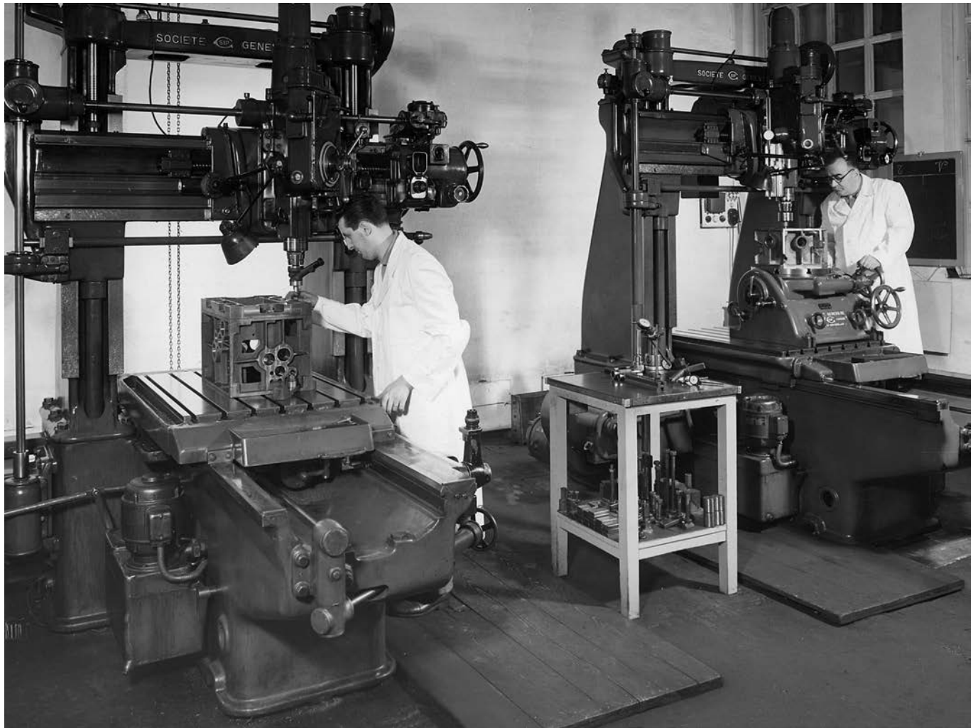
Alesatura di precisione con Genevoise in ambiente climatizzato, anni '60 Museo del Patrimonio Industriale, fondo Minganti
