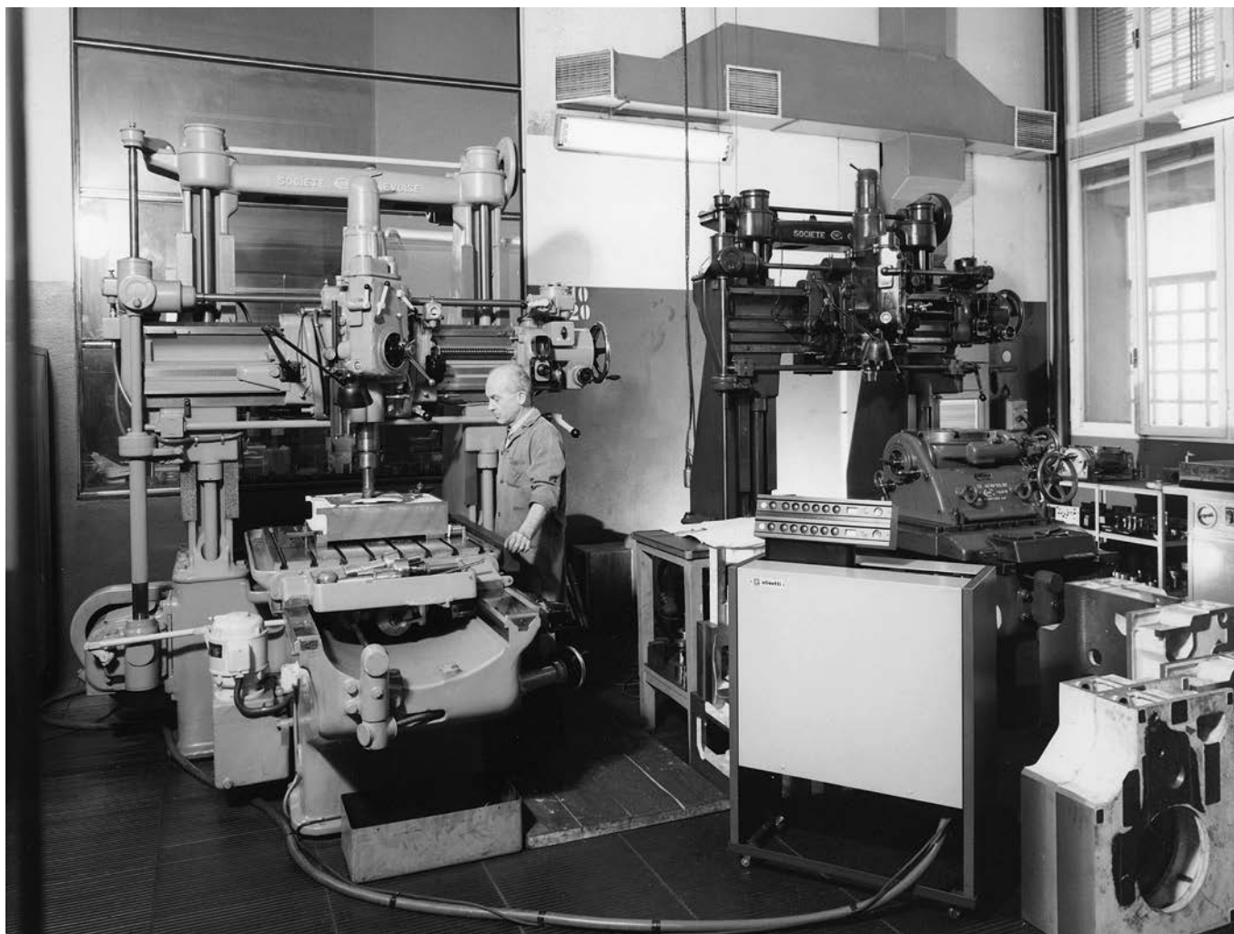
Operazione di alesatura, anni '60 Museo del Patrimonio Industriale, fondo Minganti
