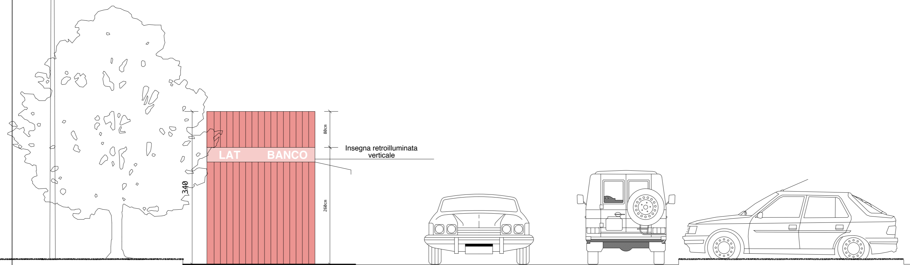
FIANCO scala 1:50
