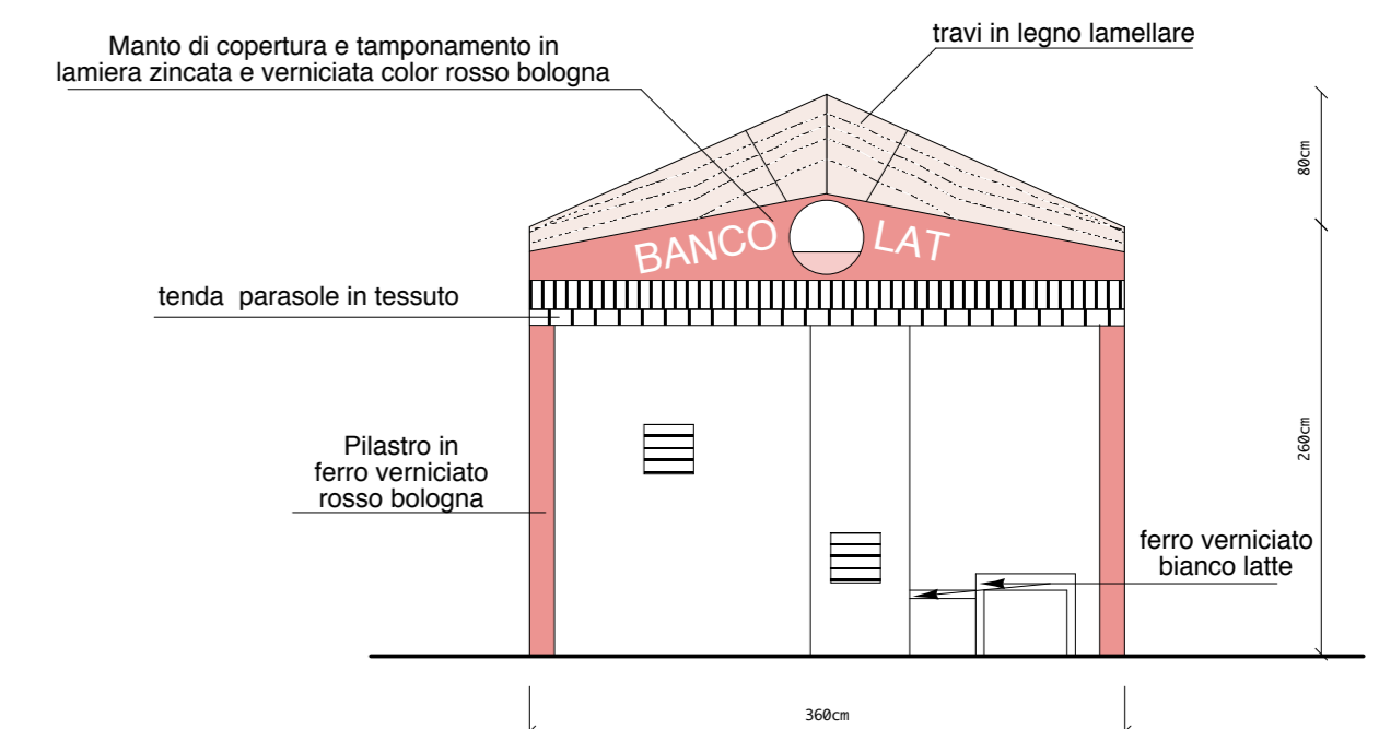
PROSPETTO scala 1:50
