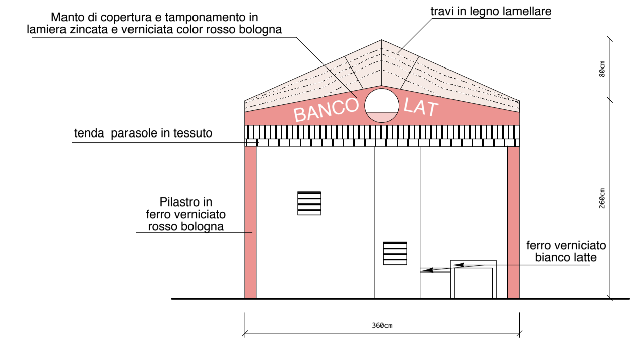
PROSPETTO scala 1:50
