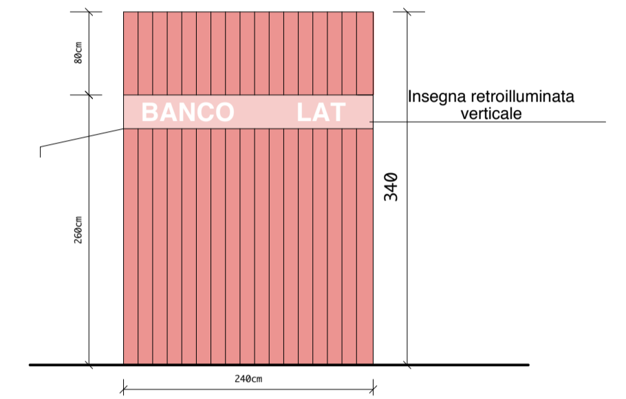
FIANCO scala 1:50
