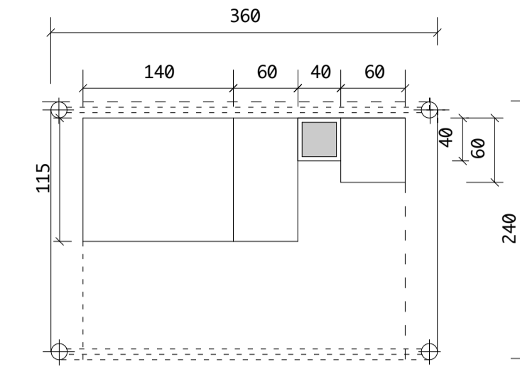
PIANTA scala 1:50
